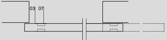
PORMENOR SUPERIOR COM RODAPE (32MM)
